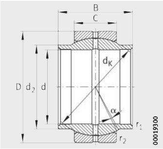
GE...LO Steel/steel
