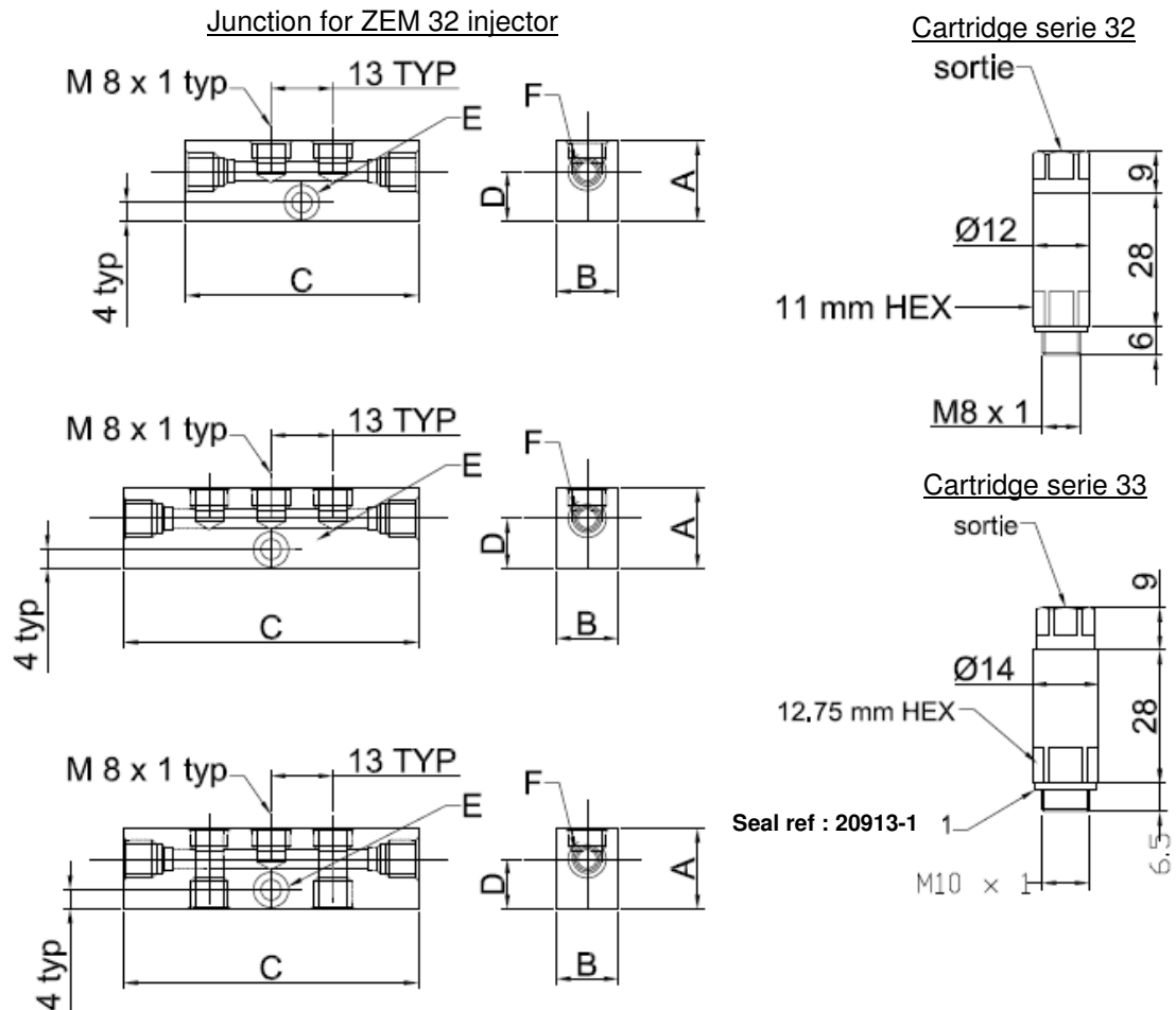
Junctions reference 32 serie
