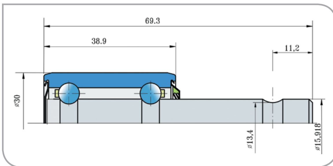
Osnovne mere/Dimensions (mm)
